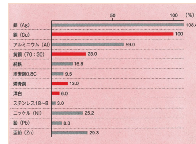
図1) 導電率
