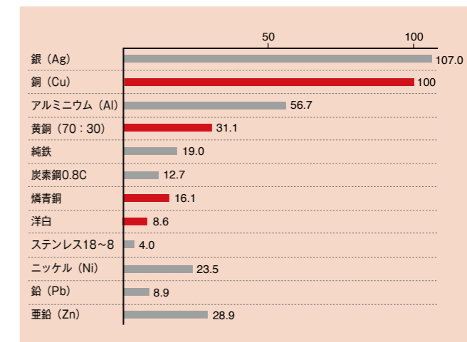
図2) 熱伝導率
